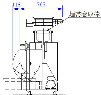
右側面図
