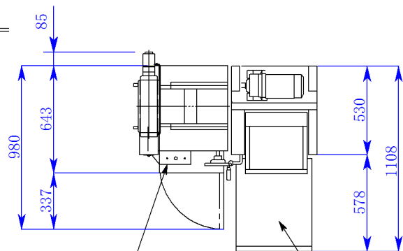
平面図
