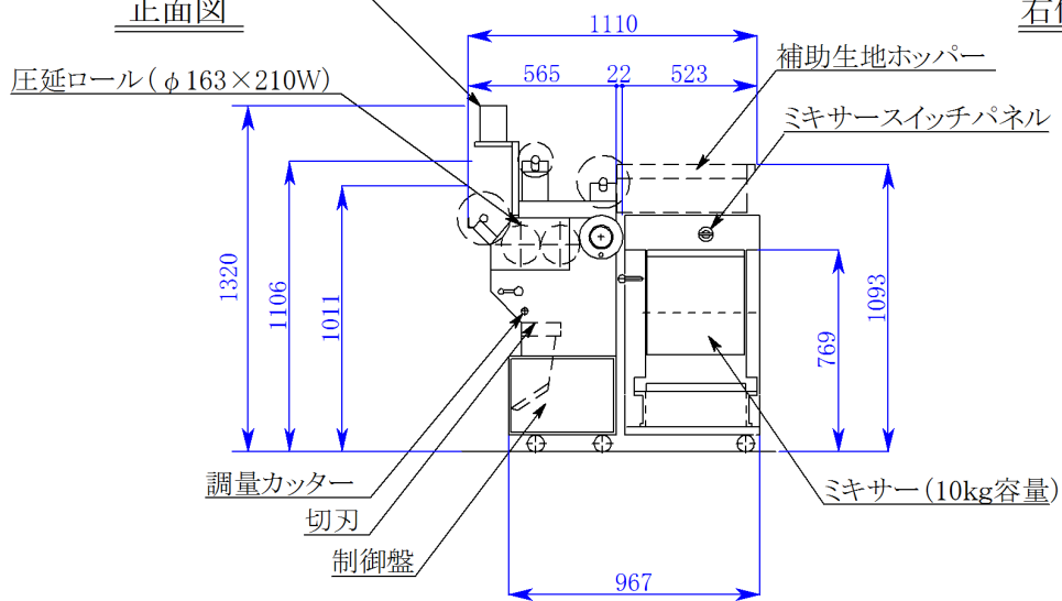
正面図
