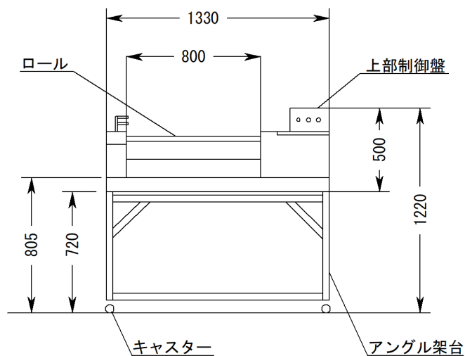
補助テーブル
