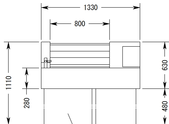
粉受けトレイ引出状態
