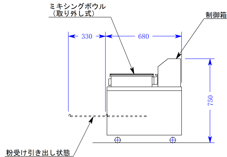
右側面図
