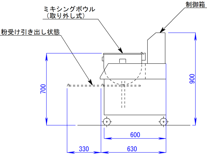
右側面図
