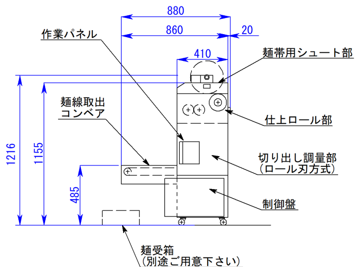
正面図
