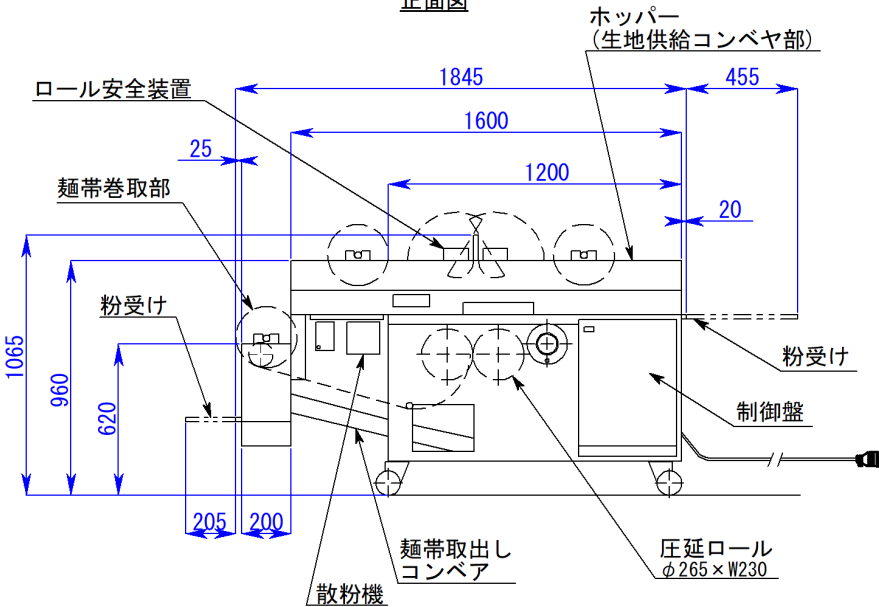
正面图
