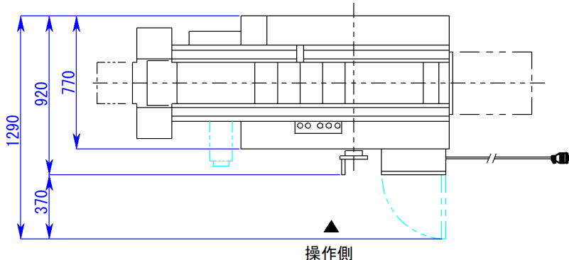
平面图
