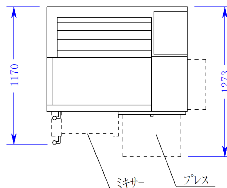
ミキサープレス引き出し時寸法
