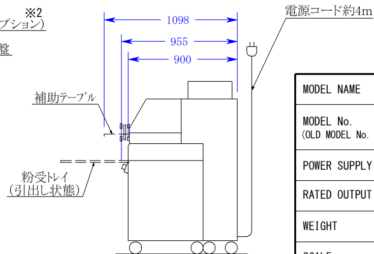
右側面図
