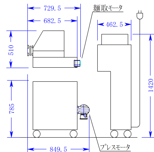
分解搬入時寸法
