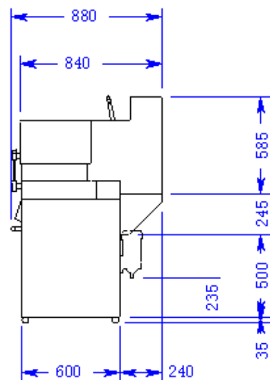
右側面図
